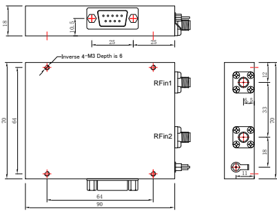
XB-17A UNIT:mm
