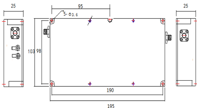
XB-2F-M UNIT: mm
